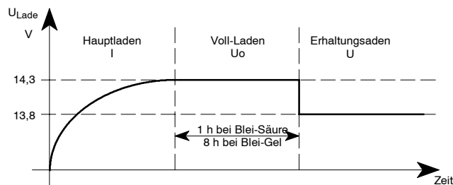
Bild 3 Beispiel für den Ladespannungsverlauf mit dem Elektroblock EBL 101 C
