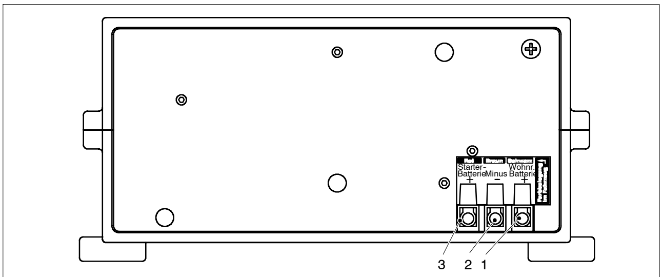
Bild 5 Aufbau Elektroblock EBL 101 C (Rückseite)
