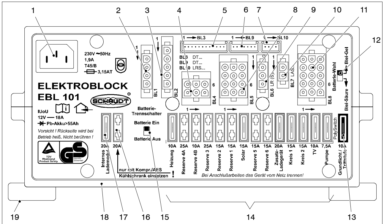
Bild 4 Aufbau Elektroblock EBL 101 C (Front)
